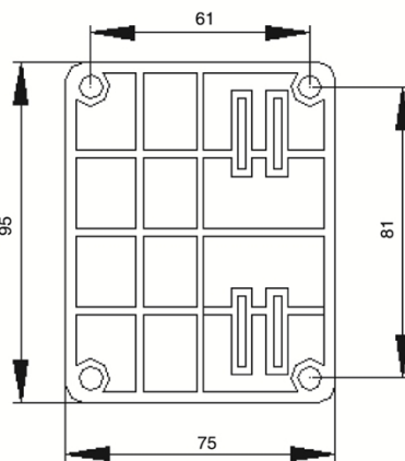
安装支架
